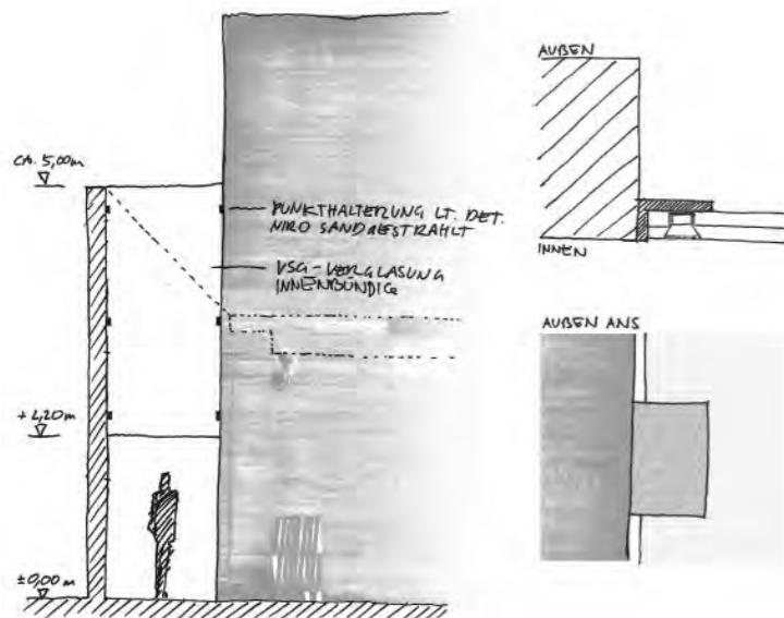
Detail Verglasung Rückseite
